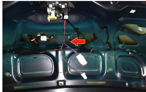
4-2. Y자 래치 케이블을 이용하여 그림과 같이 연결.
