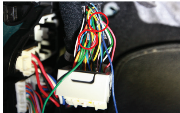
5-9. 그림과 같이 선을 연결.
