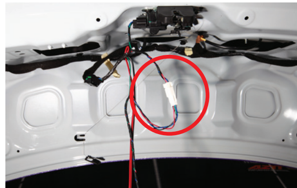
4-3. Y자형 래치 케이블에 래치 연장선 연결.
